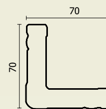
DD Уголок C1070-WG (70x70)
